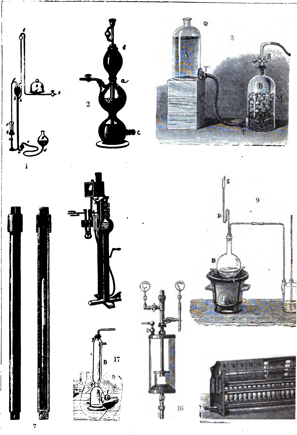
1. Ртутный насос Менгелъевъ. 2. Аппаратъ Киппа. 3. Аппаратъ С. К. Девиля. 4. Экстрактёръ Соколета-ниемъ. 7. Муфта для запаивающихъ трубокъ. 8 Ртутный насосъ Гейслера. 9. Приборъ для добыванія газовъ. Мейера для запаивающихъ трубокъ. 15. Печь для органическаго анализа. 16. Дующій насосъ Минке. 17.
